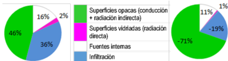
Figura 5. Distintos tipos de aporte a la carga térmica total horaria de refrigeración (izquierda) y de calefacción (derecha) de las viviendas-caso (considerando toda la vivienda climatizada).
