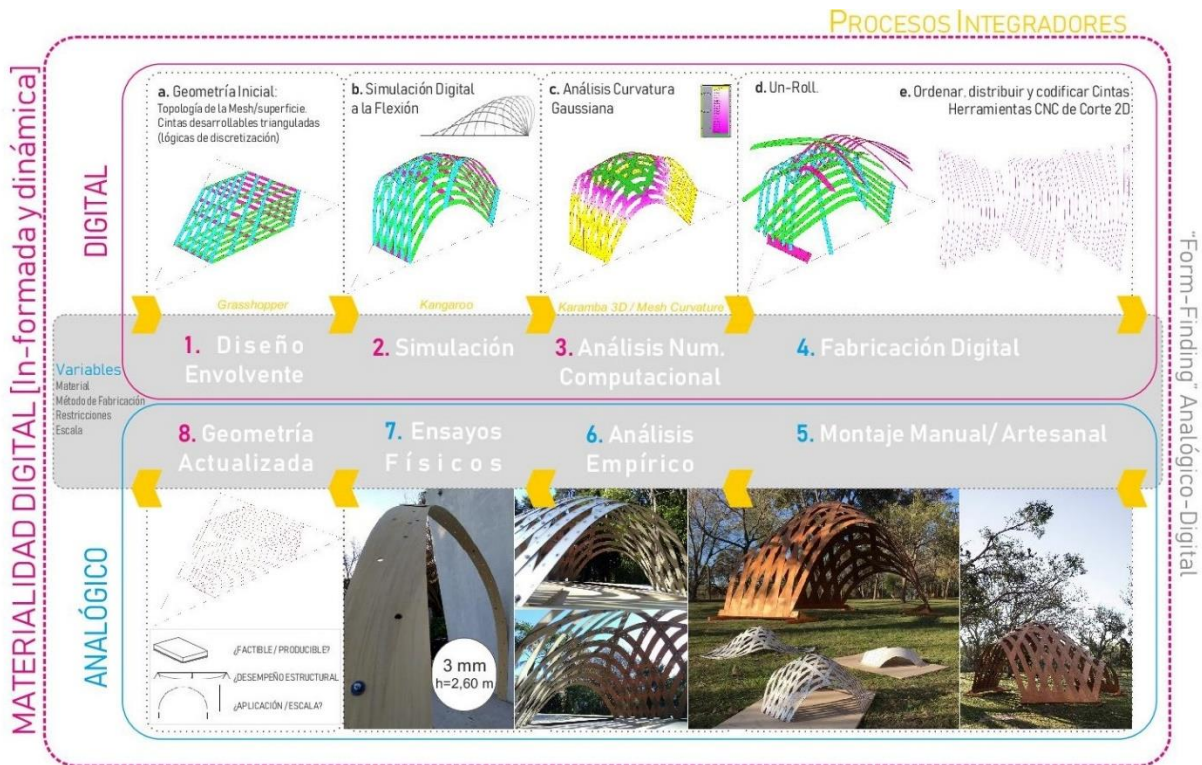
Figura 1: Procesos Integradores de diseño y construcción para envoltorios laminares a Flexión Activa. Fuente: Elaboración propia.
