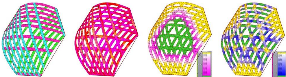
Figura 2: Simulación a flexión, Análisis de Curvatura Gaussiana y Van Mises Stress. Fuente: Elaboración propia.
