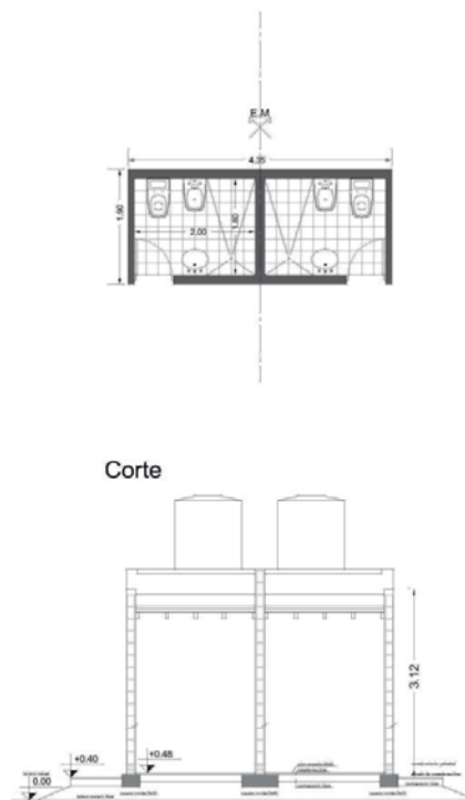
Fig.1 Planta y Corte de lo que serían en un principio dos baños apareados
