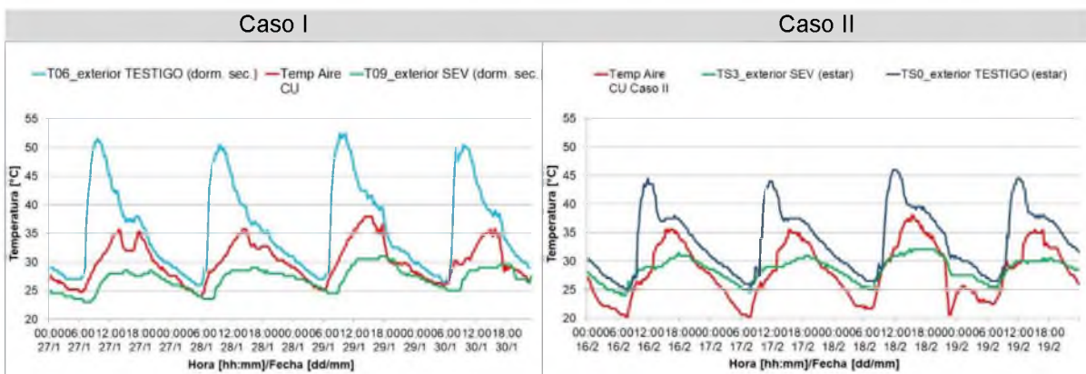
Figura 7: Diferencia de temperatura superficial exterior entre caso testigo y caso con SEV, orientación este.
