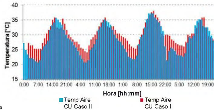
Figura 6: Temperaturas de aire exterior en el Cañón Urbano (CU) para ambos casos de estudio.
