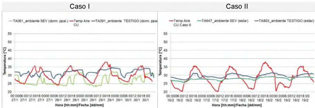
Figura 9: Diferencia de temperatura ambiente interior entre caso testigo y caso con SEV, para orientación este.
