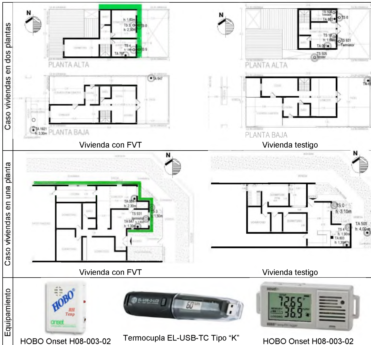
Figura 5: Plantas de las viviendas evaluadas con ubicación de sensores (color gris), y las FVT (color verde).
