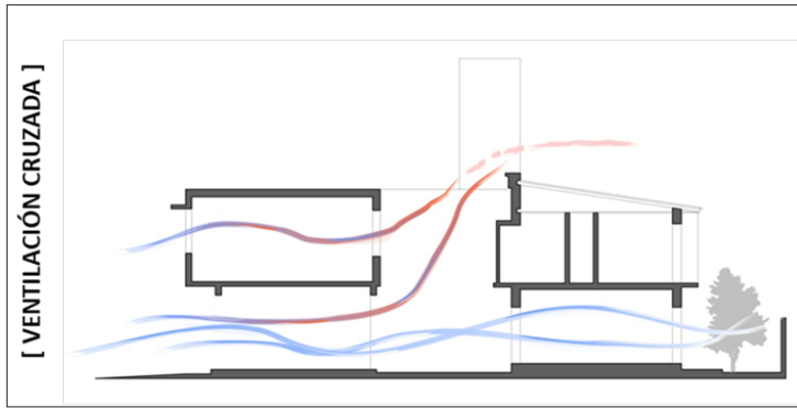
Fig. 15: Ventilación cruzada
