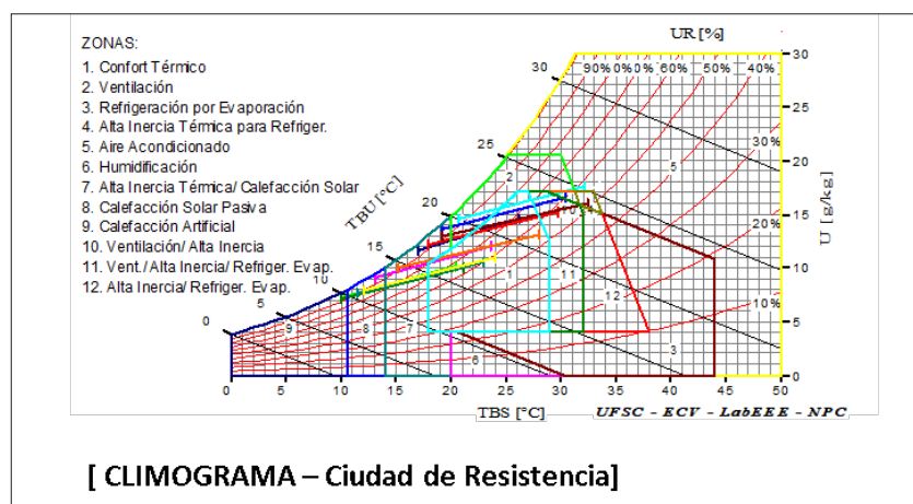
Fig. 09. Climograma. Diagrama de Givoni Ciudad de Resistencia. Fuente: autor
