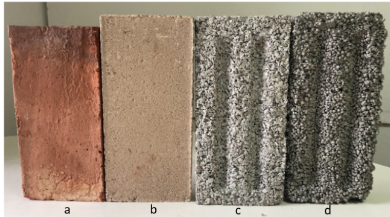
Figura 2. a) bovedilla; b) bovedilla-BTC; c) bovedilla-PET; d) bovedilla-APR.
