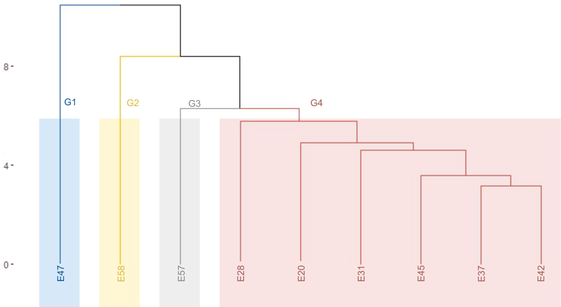
Fig. 4. Fenograma que agrupa nueve entradas de Tara spinosa , de nueve provincias de Cajamarca, caracterizadas con siete descriptores morfológicos de plántula, mediante el algoritmo k-medias, basado en la distancia euclidiana
