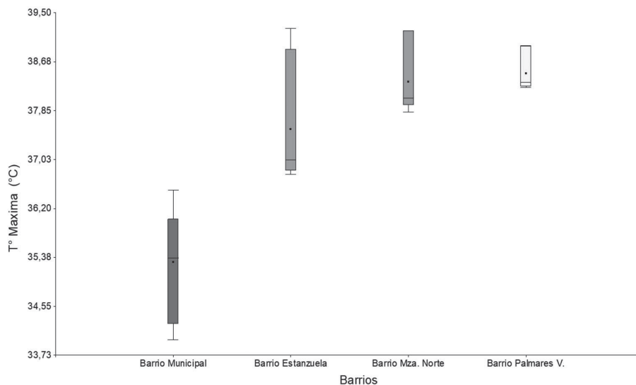
Figura 4. Gráfico box-plot para temperaturas máximas. Fuente: elaboración propia
