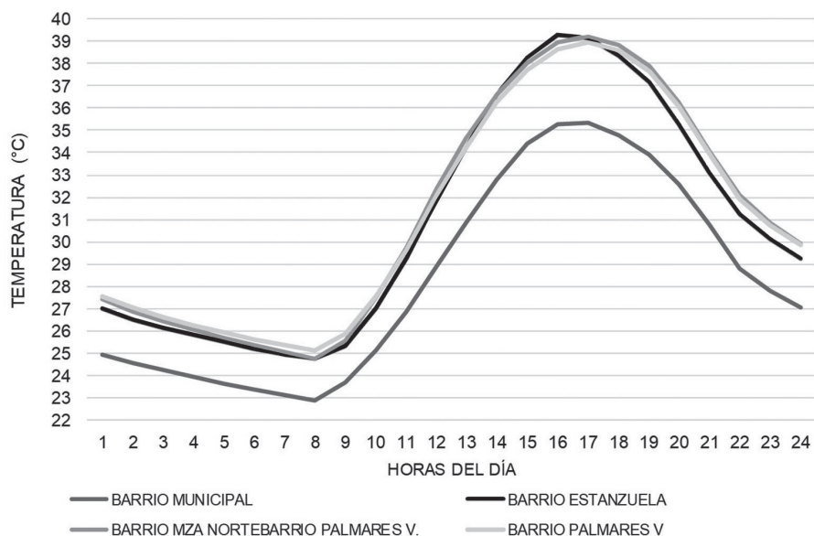
Temperaturas promedio de las propuestas analizadas
