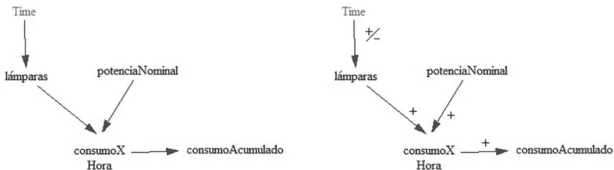
Figura 1. Modelo sistémico del consumo energético de un número de lámparas en un local (izquierda) y su diagrama de influencias (derecha)
