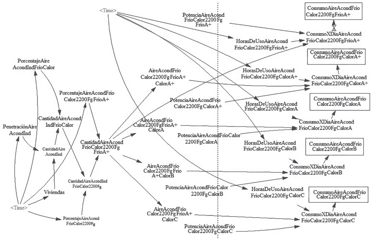
Figura 8. Parte del modelo que simula el consumo energético de los aires acondicionados frío-calor de 2200 frigorías, con etiquetado A+ para frío y sus cuatro posibles variantes para calor: A+, A, B y C
