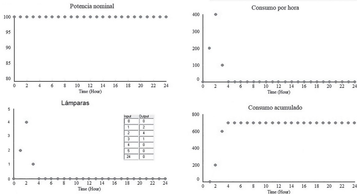
Figura 4. Evolución de las variables del sistema en función del tiempo
