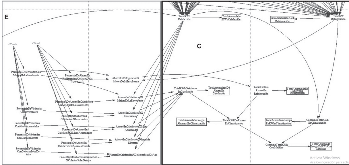
Figura 12. El bloque E modeliza las posibles medidas para ahorrar energía y el bloque C calcula los totales de consumo (diario y acumulado): por refrigeración, por calefacción y aplicando medidas de ahorro
