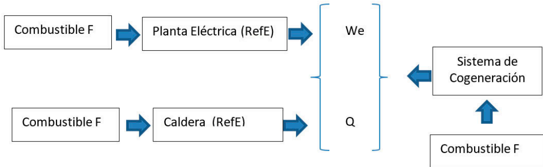
Figura N° 2 Concepto de Cogeneración versus la generación individual de calor y energía eléctrica. Dónde: Energía asociada al combustible= F , Rendimiento eléctrico \eta_e = W_e/F , Rendimiento térmico \eta_t = Q/F , Rendimiento energético = (W_e+Q)/F , Relación r = W_e/Q .
