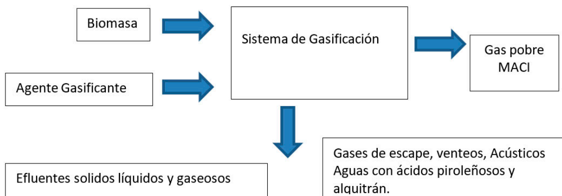
Figura N°4 Los efluentes en el proceso de gasificación. (Gráfico del proceso)
