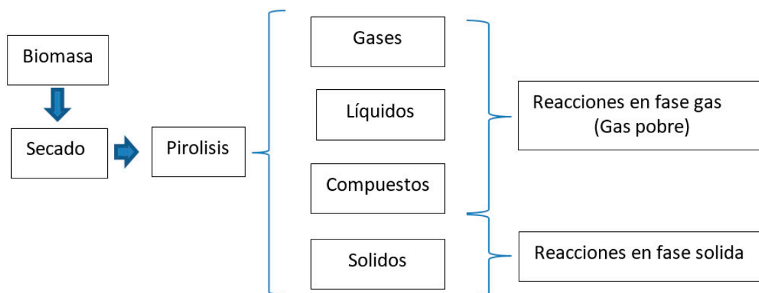
Figura N° 1 Esquematización del proceso y las rutas de reacción en la gasificación.
