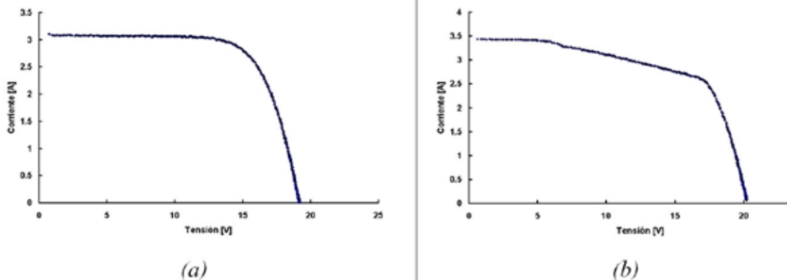
Figura 2: (a) Curva I-V de un módulo de 50 W p de correcto funcionamiento. (b) Curva I-V de un módulo de 50 W p , que presenta defectos debido a posible defecto en sus celdas componentes.
