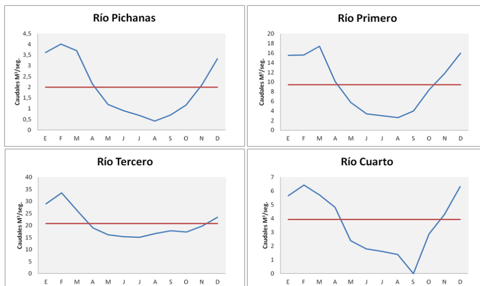
Figura N° 10. Hidrogramas de Caudales Absolutos (1961-1970).
