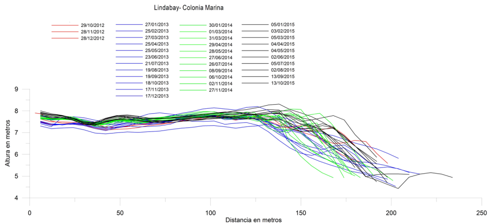
Figura 8. Perfiles de Lindabay registrados entre 2012 y 2015.
