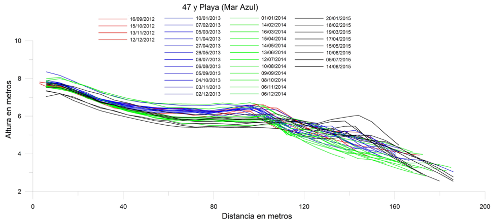
Figura 5. Perfiles de 47 y playa registrados entre 2012 y 2015.
