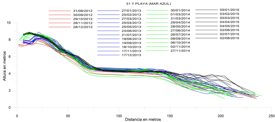
Figura 7. Perfiles de 31 y playa registrados entre 2012 y 2015.
