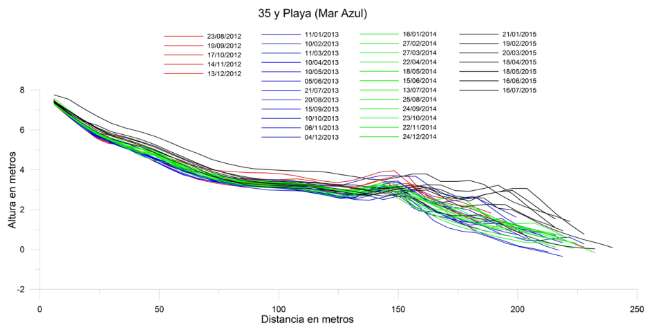
Figura 6. Perfiles de 35 y playa registrados entre 2012 y 2015.
