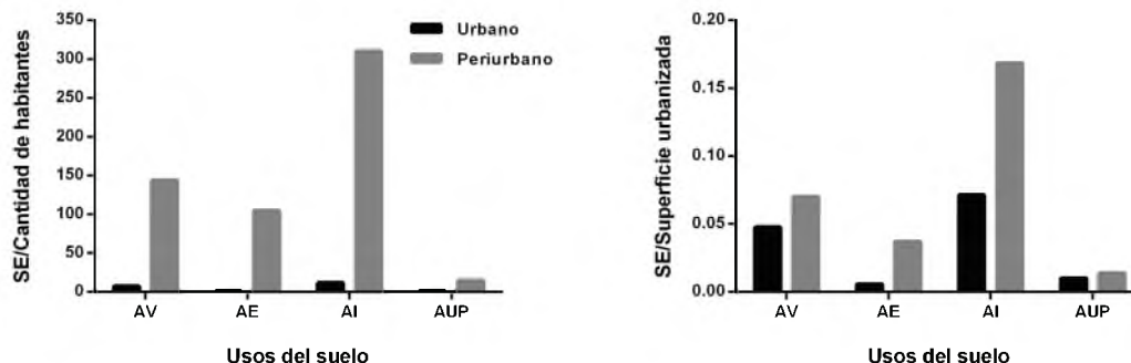
Figura 2. Relación entre A) servicios de los ecosistemas y cantidad de habitantes (millones) y B) servicios de los ecosistemas y superficie urbanizada (km 2 ) considerando cada uso del suelo (AV, AE, AI, AUP) y nivel de urbanización (urbano y periurbano). Referencias: AV: área verde, AE: agropecuario extensivo, AI: agropecuario intensivo, AUP: agricultura urbana y periurbana
