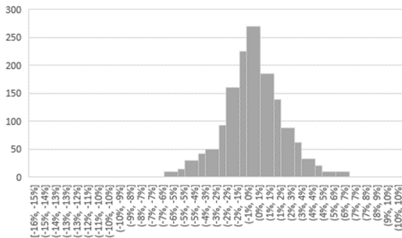
Gráfico 3. Histograma de la distribución de retornos observada
