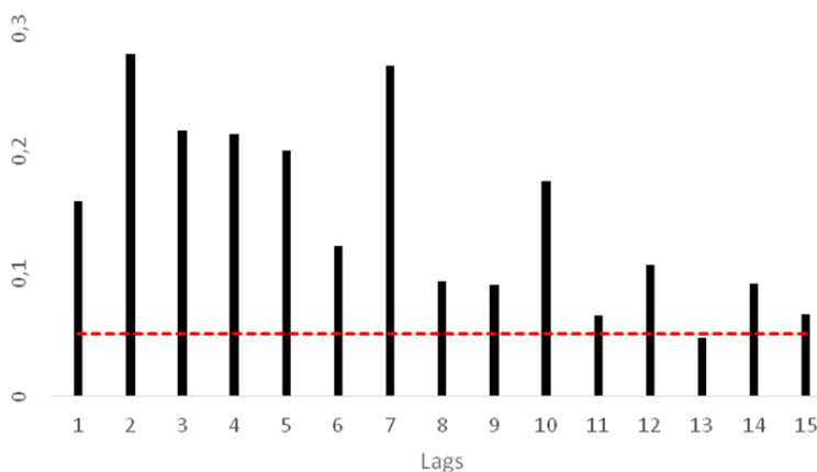
Gráfico 4. Función de Autocorrelación
