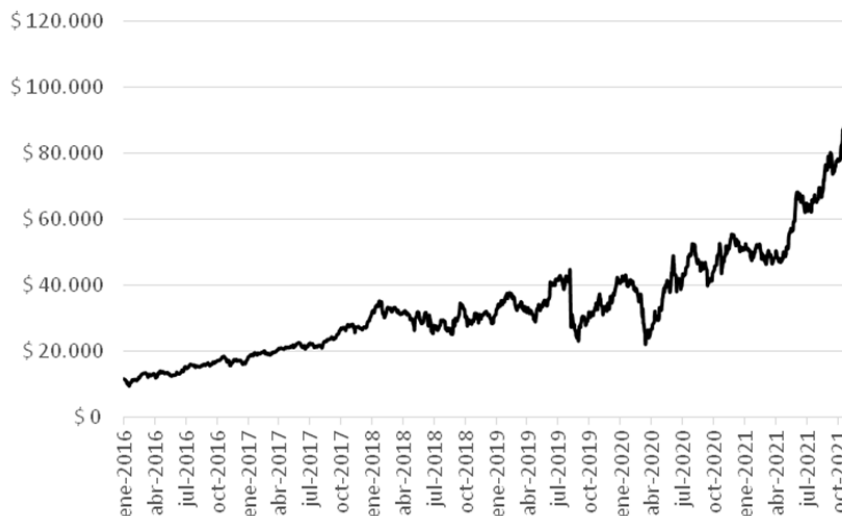
Gráfico 1. Serie diaria del Índice S&P Merval
