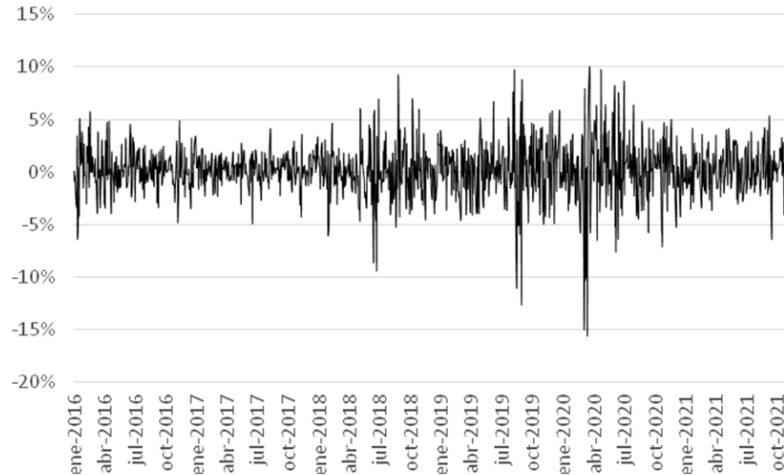
Gráfico 2. Distribución de los retornos diarios
